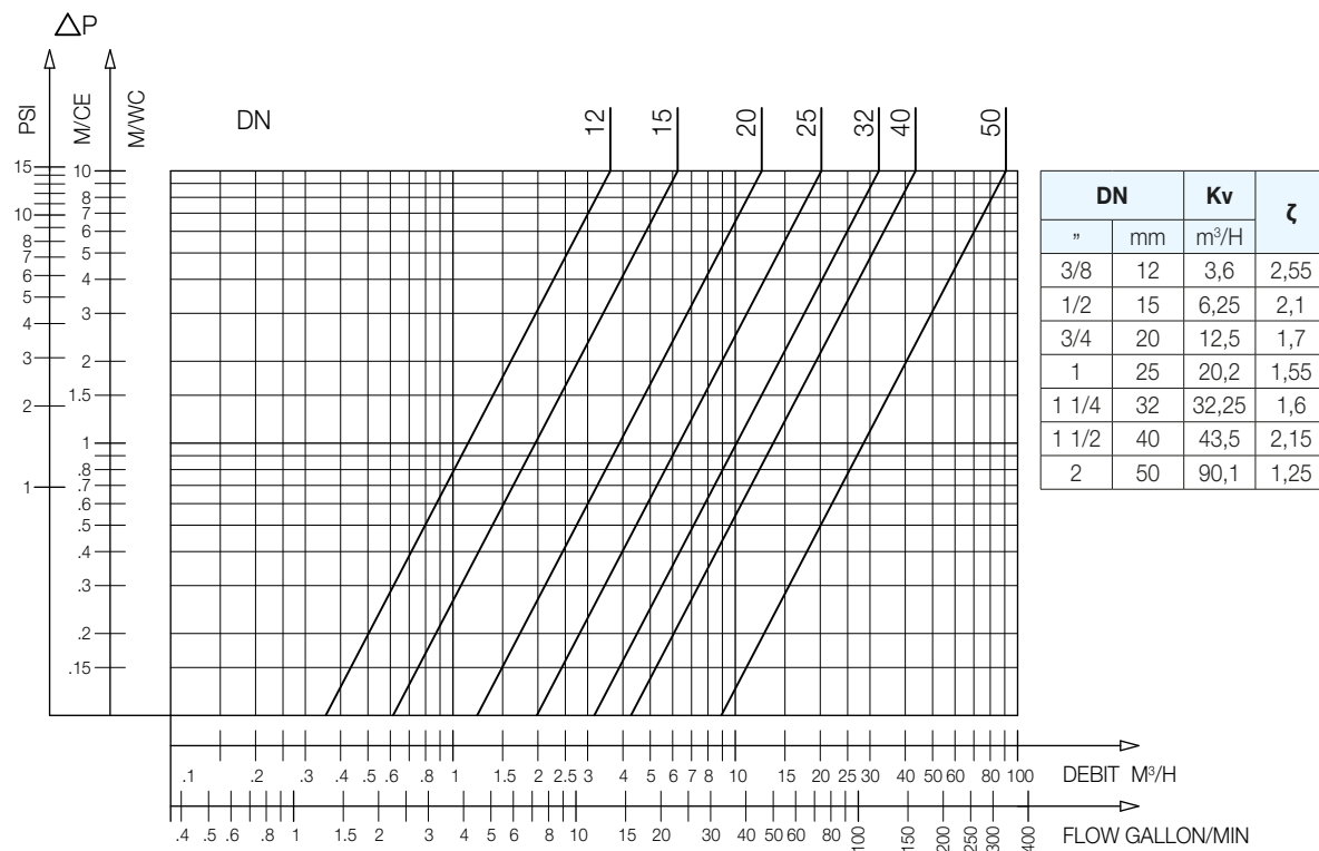
101 - Abaque des pertes de charge
